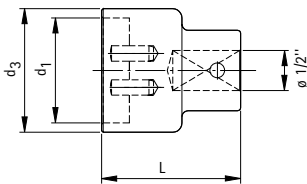
KSアセンブリレンチ
