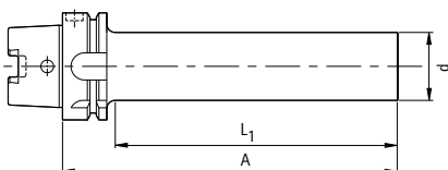
テストピン HSK-A
