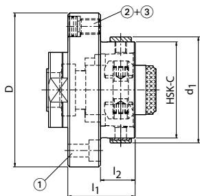
MN5000-14準拠の振れおよび倒れ調整機能付きKSフランジアダプター用スペアパーツ
