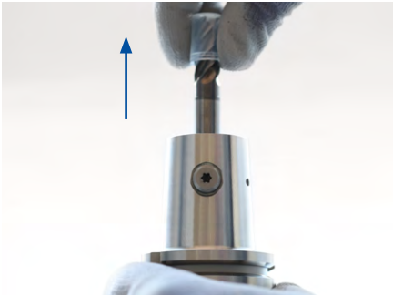
2. サーフেসチャックのロケーションボーリングからツールを取り外します。
