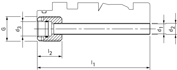
ミスト供給の連結穴を持つチューブアダプタ
