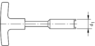
クーラントパイプもしくはKS-MMSクランピングカートリッジの受接管の取付けおよび取外し用の取付けキー
