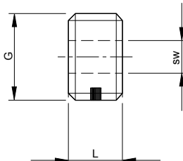
ブラインドスクリュー
