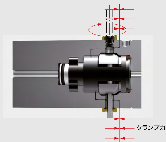
接触面とテーパのクランプありの接続
