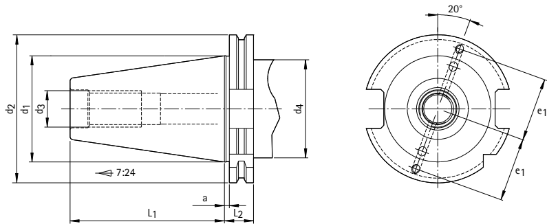
自動ツール交換用 形状 A、形状 AD、形状 AF およびデータキャリア付き仕様
