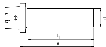
テストピン HSK-C
