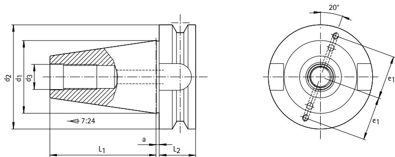
自動ツール交換用 形状 A、形状 JF、形状 JD およびデータキャリア付き仕様
