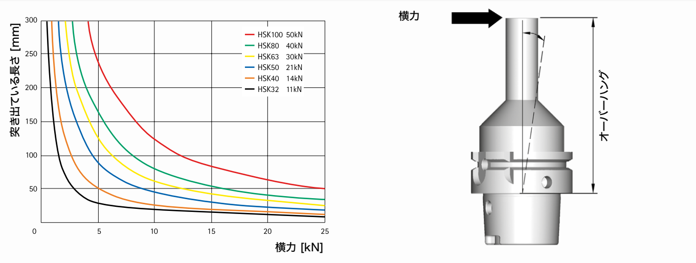
KSカートリッジ使用時のHSKインターフェースの許容曲げ荷重
