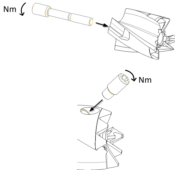
Bild 18, Gewindestift und Differentialschraube für TTS-Trennstelle
