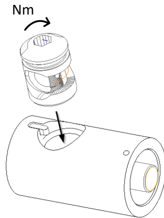
Bild 16, Exzenterbolzen für Radialspannung
