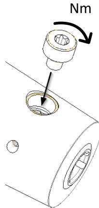
Bild 26, Spannschraube für MillChuck System-HB
