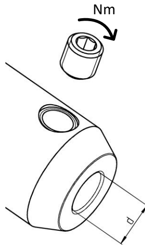
Bild 27, Spannschraube DIN1835
