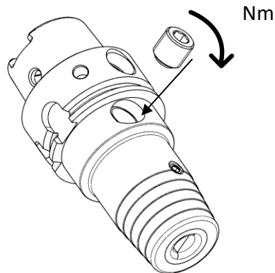
Bild 23, Gewindestift für Dehnspannaufnahmen
