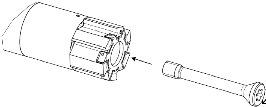
Bild 17, PSS-Trennstelle
