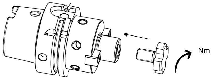
Bild 8, Fräsdornaufnahme
