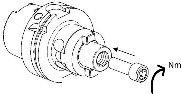
Bild 10, Zylinderschraube mit Innensechskant
