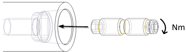
Bild 15, Gewindespindel für Axialspannung
