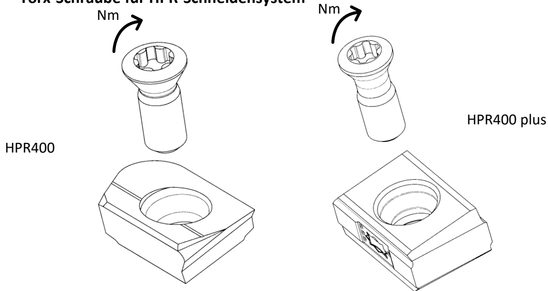
Bild 2, Torx-Plus Schraube für HPR-Schneidensystem
