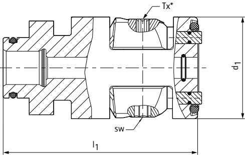
Cartuchos de sujeción KS con junta tórica exterior: versión MQL1 para HSK-A y HSK-C
