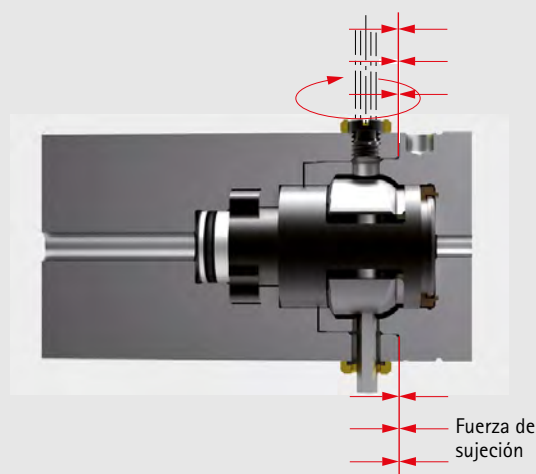
Unión sujeta de la cara plana de apoyo y el cono
