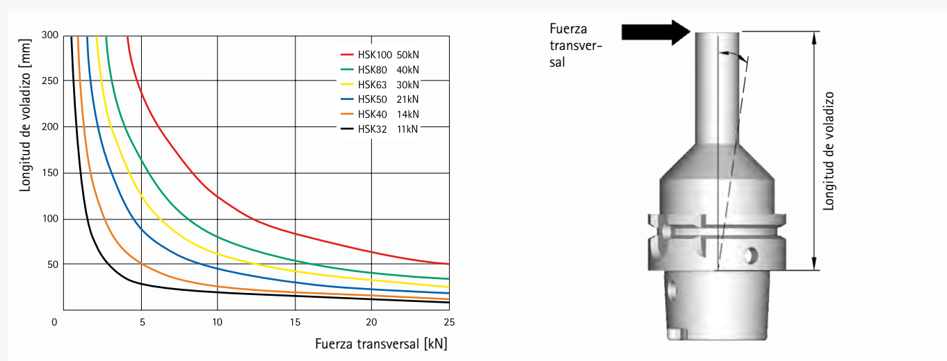
Carga de flexión admisible de la interfaz HSK cuando se utilizan los cartuchos KS
