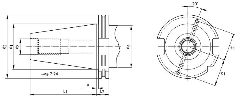
Para cambio de herramienta automático, forma A, forma AD, forma AF y ejecución con soporte de datos
