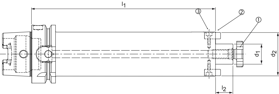
Para portafresas con diámetro del apoyo ampliado según DIN 69882-3
