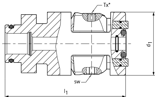
Cartuchos de sujeción KS con junta tórica interior: versión MQL para HSK-A y HSK-C
