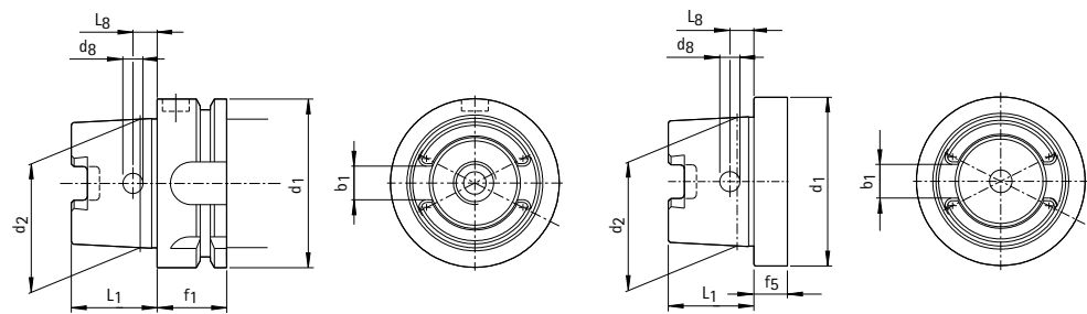
HSK-A para el cambio automático y manual de herramienta
