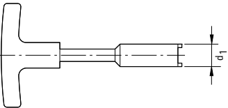
Llave para el montaje y desmontaje de tubos de refrigerante o de tubos adaptadores de los cartuchos de sujeción KS MMS
