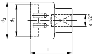
Llaves de vaso de montaje KS
