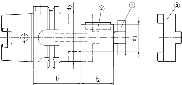
Para portafresas, para fresas con ranura longitudinal/transversal según DIN 69882-2
