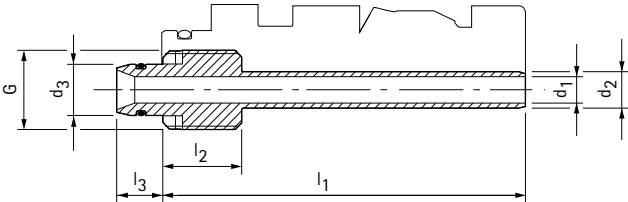
Tubos adaptadores con conexión de pivote
