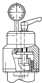
Calibres de medición para chaflanes de sujeción de 30°
