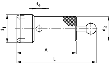
Pinzas de montaje KS para aplicaciones MMS
