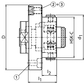
Refacciones para brida antepuesta KS con alineación radial y angular según MN 5000-14
