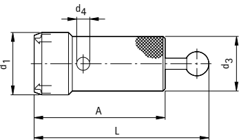
Pinzas de montaje KS
