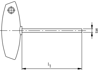
Destornillador hexagonal con mango en T
