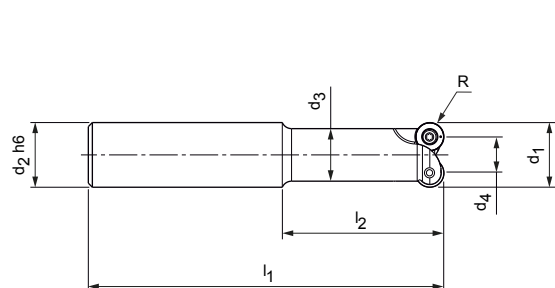
Fresa di finitura, versione cilindrica
