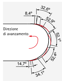
Avvolgimento a seconda del percorso di posizionamento – curva della traiettoria ottimizzata
