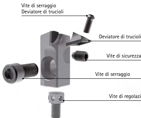
Cartuccia di fresatura Power (PMC)
