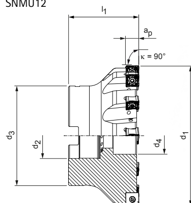
Fresa a manicotto, passo medio
