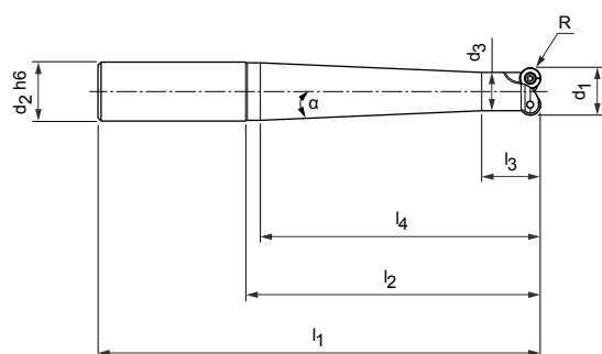
Fresa di finitura, versione conica
