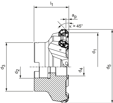
Fresa a manicotto, passo stretto
