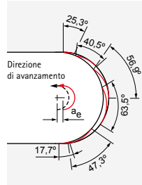
Avvolgimento a seconda del percorso di posizionamento – traiettoria circolare
