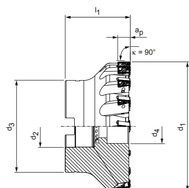
Fresa a manicotto, passo medio
