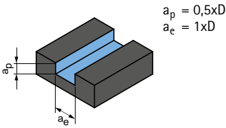
Fresatura di scanalature
