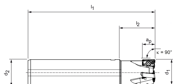
Fresa di finitura
