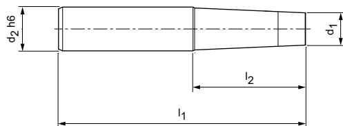
Konische Ausführung aus Stahl, CFS201 | Lagerhaltige Vorzugsbaureihe
