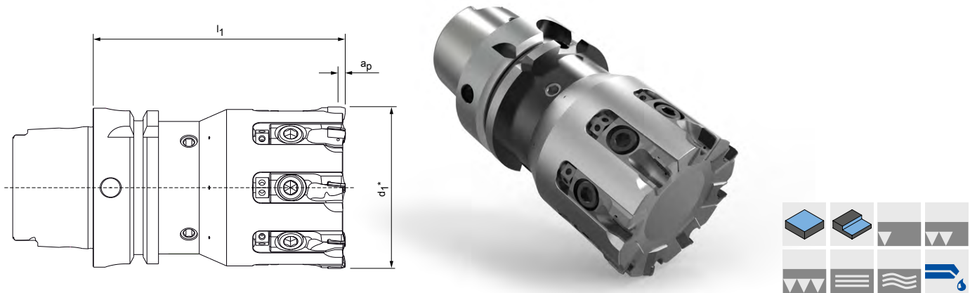
Corps de base avec interface HSK-A
