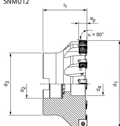
Fraises à axe horizontal, division standard
