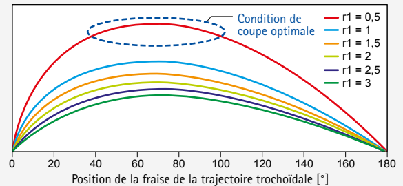
Contact dépendant de la trajectoire et de son rayon
