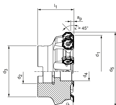
Fraises à axe horizontal, division standard
