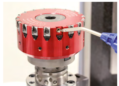
3. Nettoyer le logement de l'insert de fraisage avec de l'air comprimé puis introduire par le haut le nouvel insert de fraisage dans le guidage en queue d'aronde.
