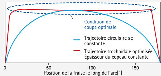
Contact dépendant de la trajectoire – trajectoire circulaire conventionnelle et trajectoire optimisée
