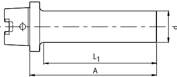
Prüfdorne HSK-C
