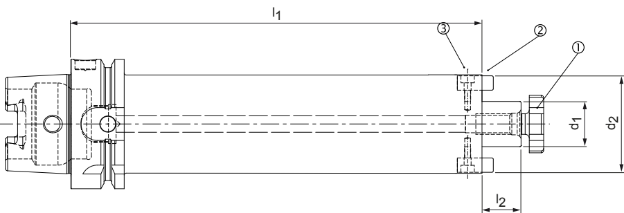
Für Aufsteckfräserdorne mit vergrößertem Anlagedurchmesser nach DIN 69882-3
