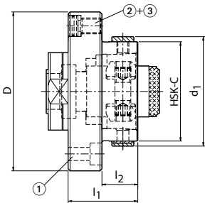
Ersatzteile für KS-Vorsatzflansch mit Radial- und Winkelausrichtung nach MN 5000-14
