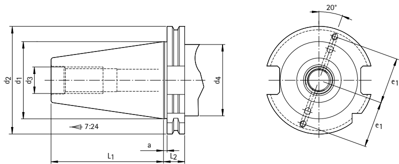
Für automatischen Werkzeugwechsel Form A, Form AD, Form AF und Ausführung mit Datenträger
