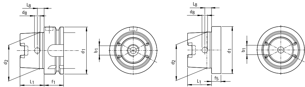
HSK-A für automatischen und manuellen Werkzeugwechsel
