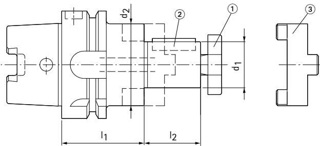
Für Aufsteckfräserdorne für Fräser mit Längs-/Quernut nach DIN 69882-2
