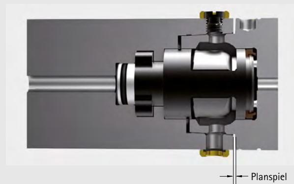
Ungespannte Plananlage-Kegel-Verbindung
