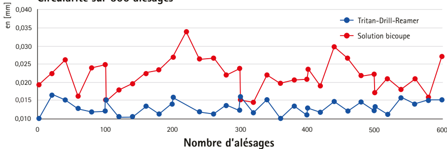
Circularité sur 600 alésages
