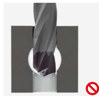
Perçage centré et \gg D
