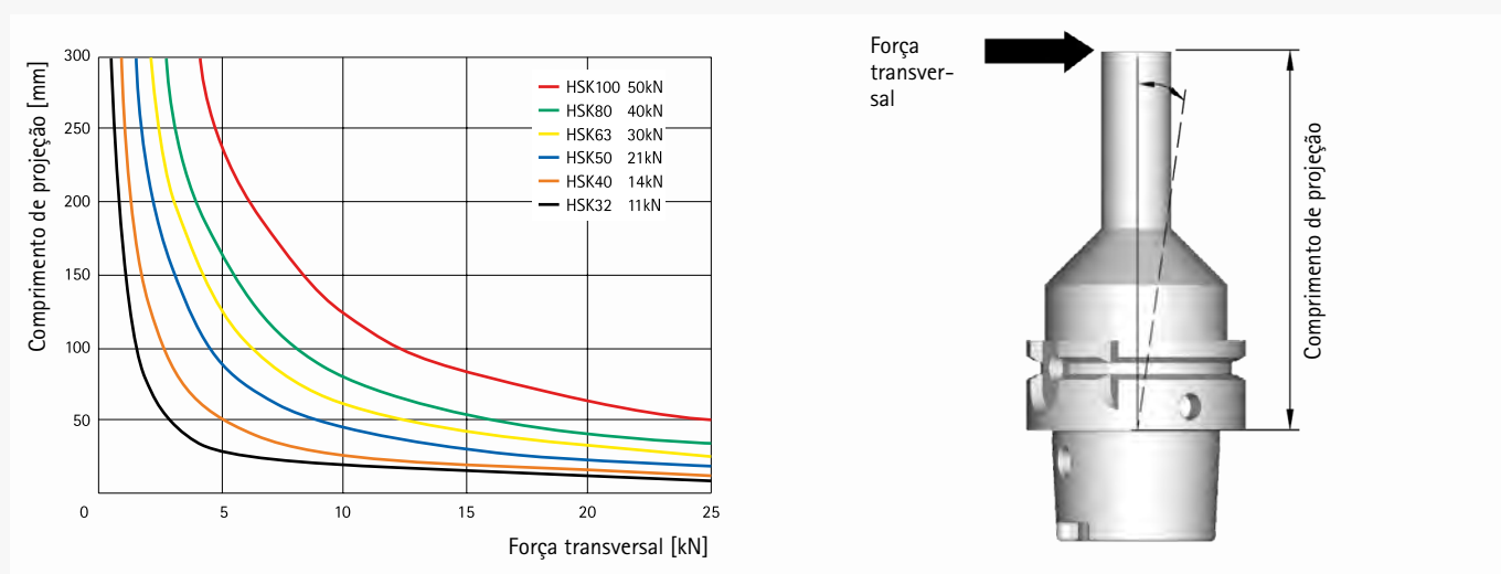
Sobrecarga de flexão permitida da interface HSK quando do uso do cartucho KS
