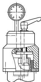
Calibres para 30° de inclinação de fixação
