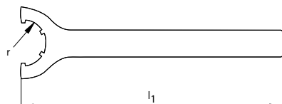
Chave de fixação para suporte para pinças de fixação conforme DIN 69882-6 e mandril rosqueado Softsynchro
