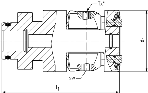
Cartuchos de fixação KS com Anel em O externo – versão MQL1 para HSK-A e HSK-C
