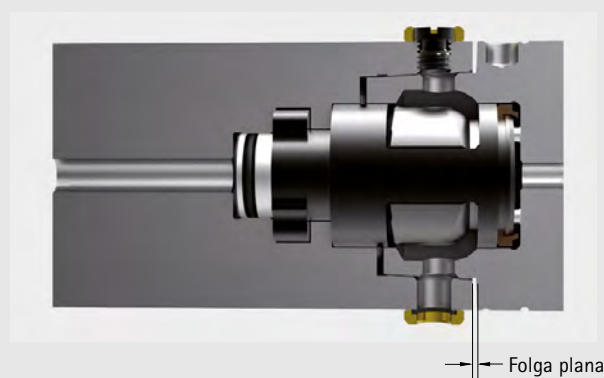
União do cone de face plana não tensionada
