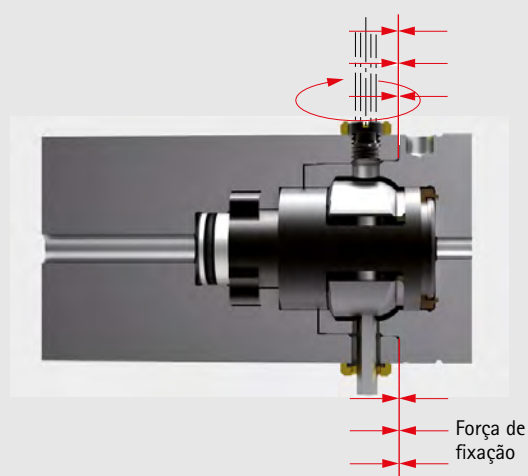
Ligação cone-equipamento plano fixada
