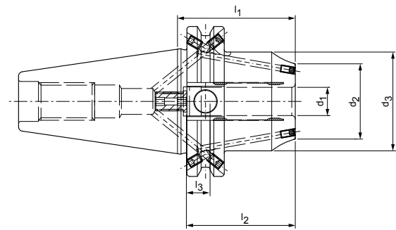
Modelo curto pesado com dois orifícios de canal de refrigeração, reutilizável
