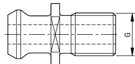
Pino de aperto para cone de grande abertura conforme ASME B 5.50 (CAT)
