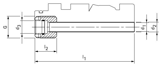
Tubo adaptador com transição de perfuração
