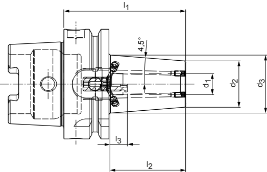
Modelo com dois furos de canal de refrigeração que podem ser fechados novamente
