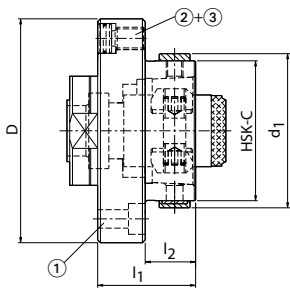
Peças sobressalentes para flange de guarda KS com alinhamento radial e angular conforme MN 5000-14
