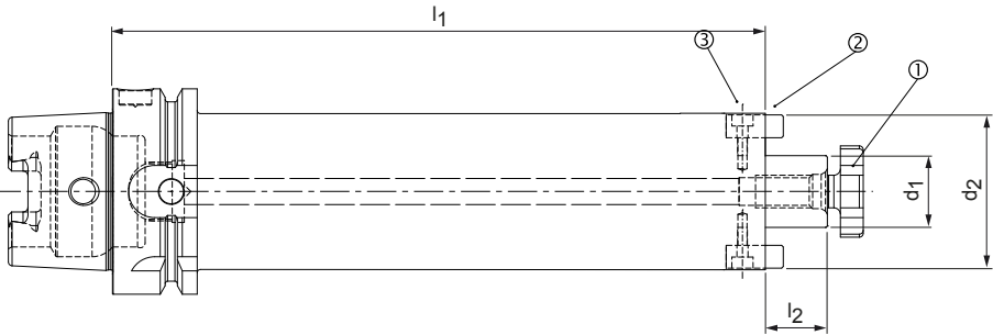
Para mandris porta-fresas de encaixe com diâmetro de encosto aumentado de acordo com DIN 69882-3
