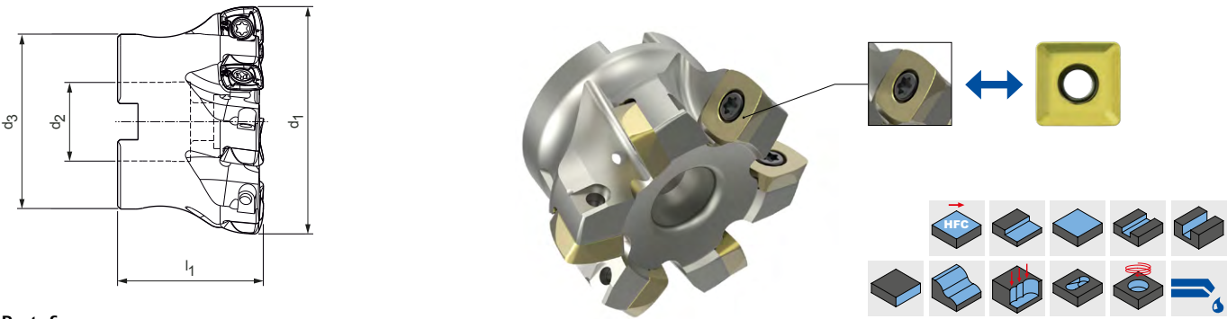
Portafresa
