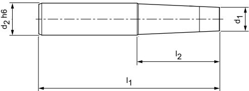
Ejecución cónica de acero, CFS201 | Serie preferente disponible en stock
