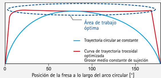
Enlazado en función de la posición de trayectoria: trayectoria circular convencional y curva de trayectoria optimizada
