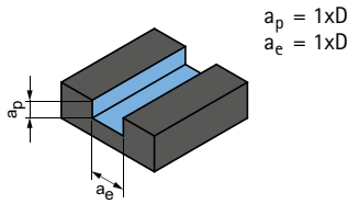
Fresado de ranuras
