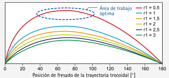
Enlazado en función de la posición y el radio de la trayectoria
