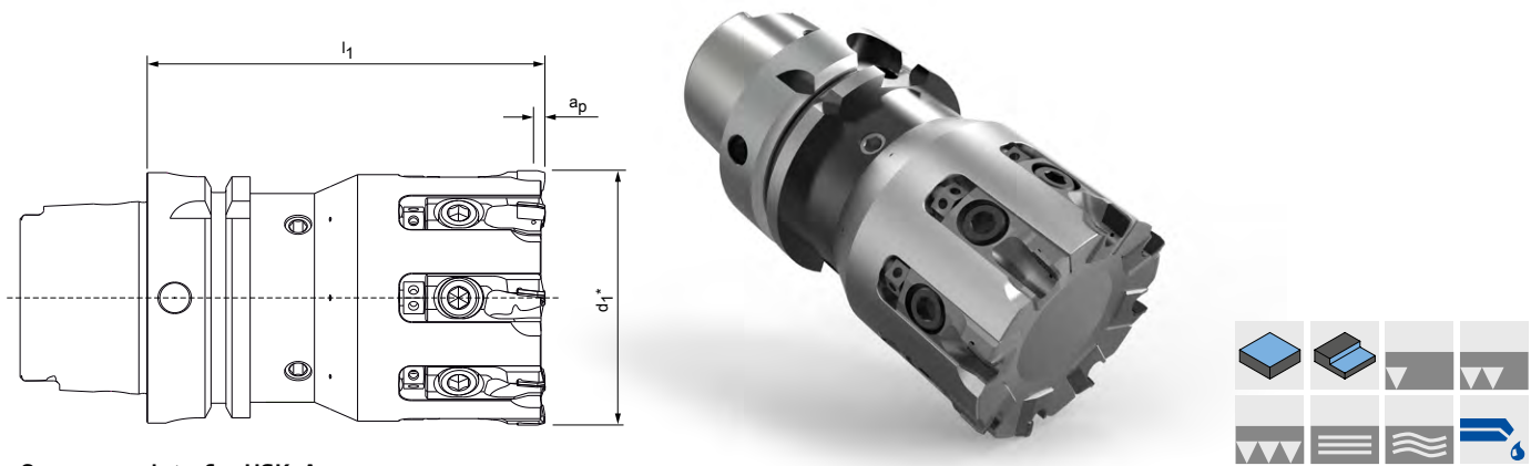
Cuerpo con interfaz HSK-A
