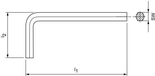
Destornillador acodado hexagonal
